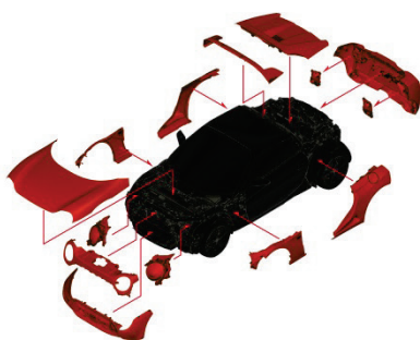
「S660 Neo Classic KIT」 外装、灯体組替パーツイメージ
